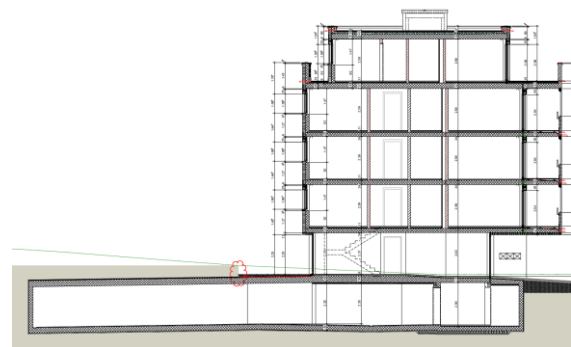
Gebäudeschnitt
