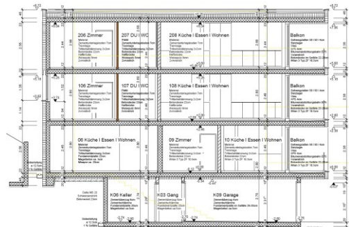
Gebäudeschnitt
